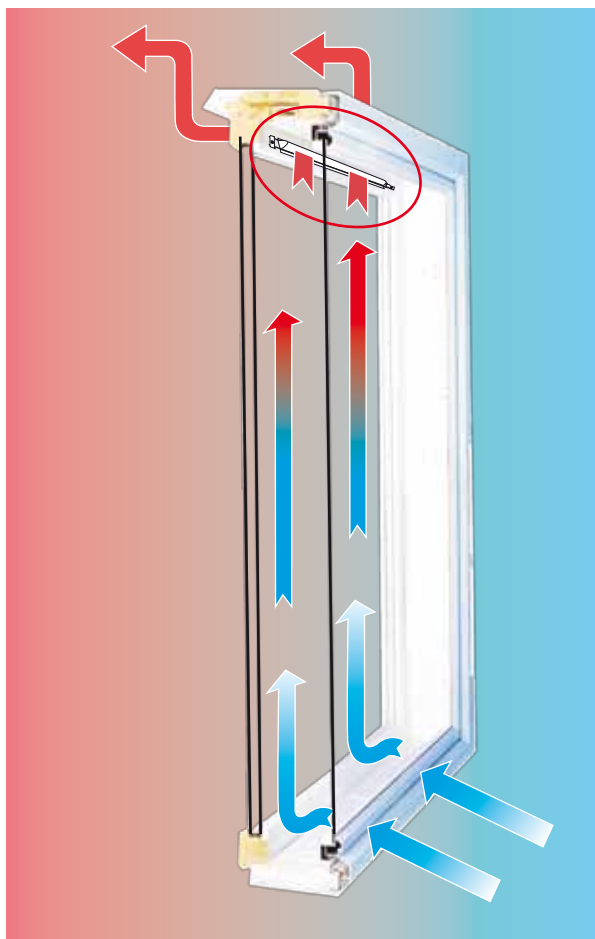
Asennettu rakoventtiili
